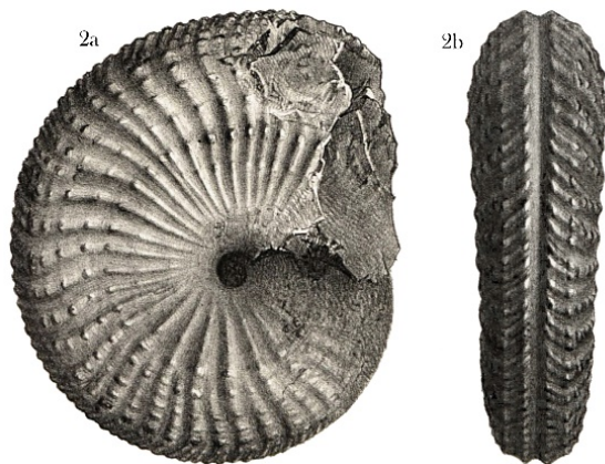
Abb. 2.15: Sirenites argonautae (Holotyp, MOJISOVICS 1893: Taf. CLVI, Fig. 2a,b)
